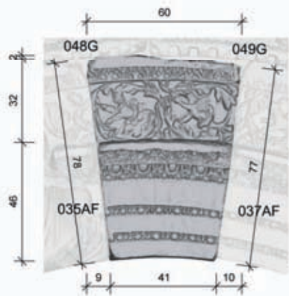
Ansicht Süd
