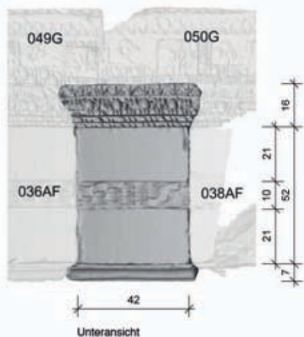
Unteransicht
