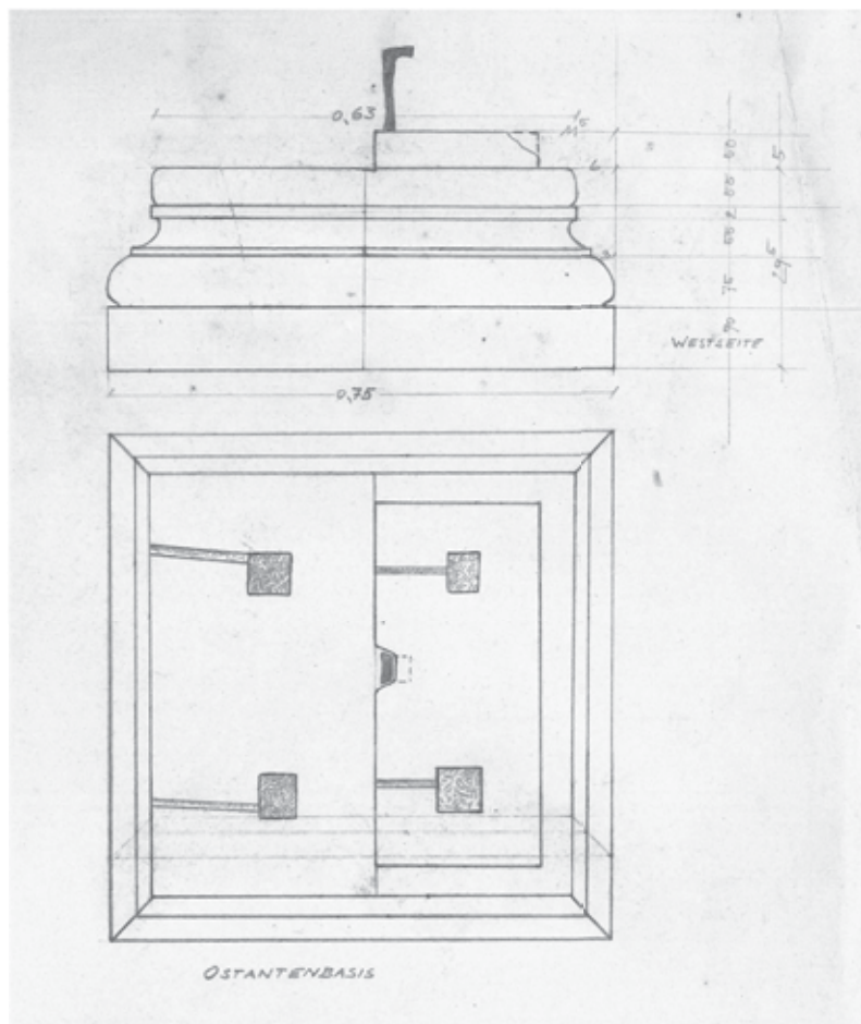
2 Pfeilerbasis 023B (Zeichnung K. H. Göschl)
