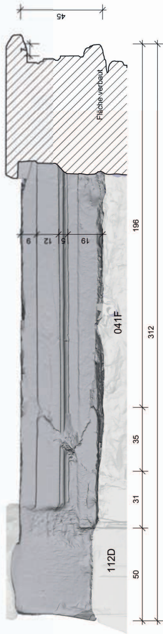
Rückseite
