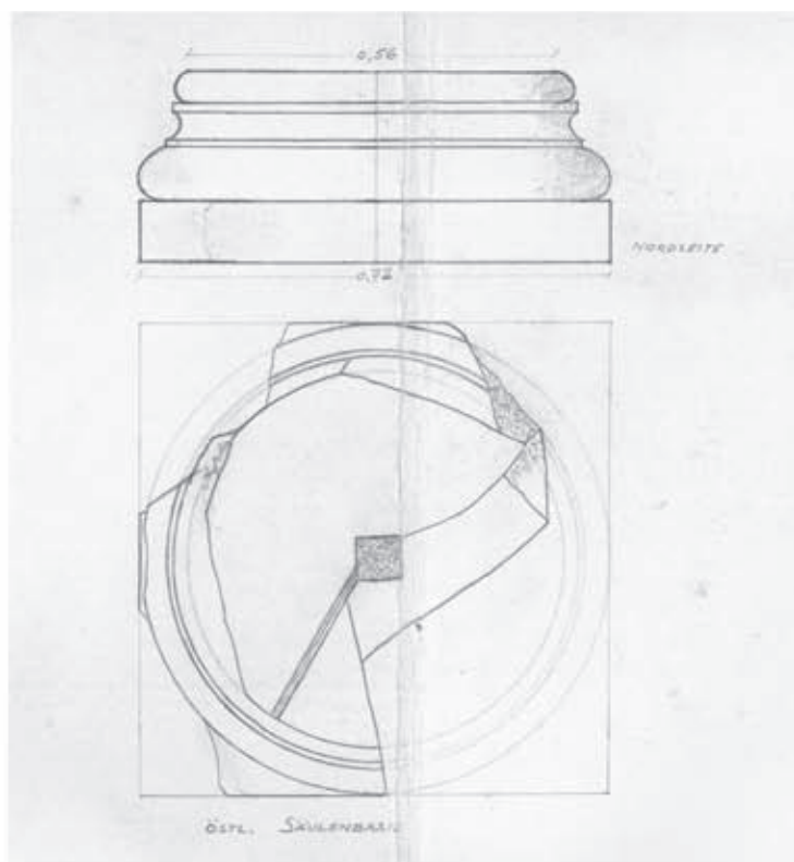
1 Verschollene Säulenbasis 171B (Zeichnung K. H. Göschl)
