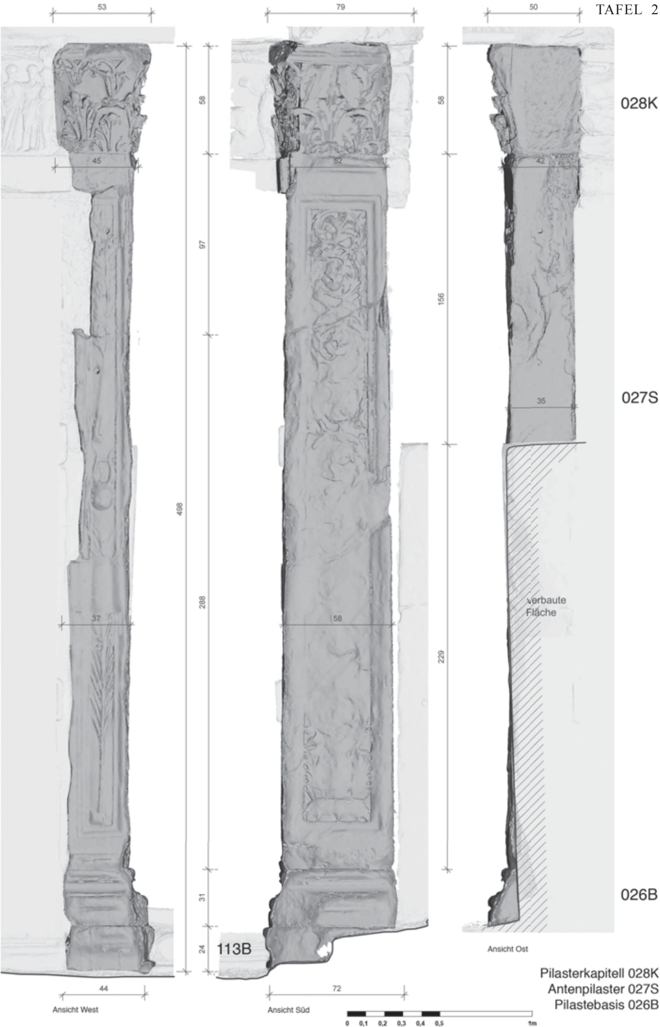
Pilasterkapitell 028K, Antenpilaster 027S sowie Pilasterbasis 026B
