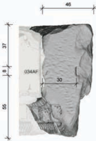
Stoßfläche West
